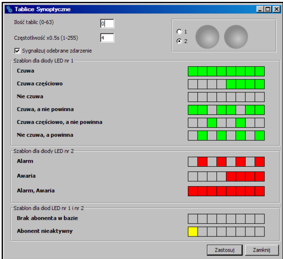
Rys. 33. Okno „Tablice synoptyczne” po pierwszym uruchomieniu programu.
